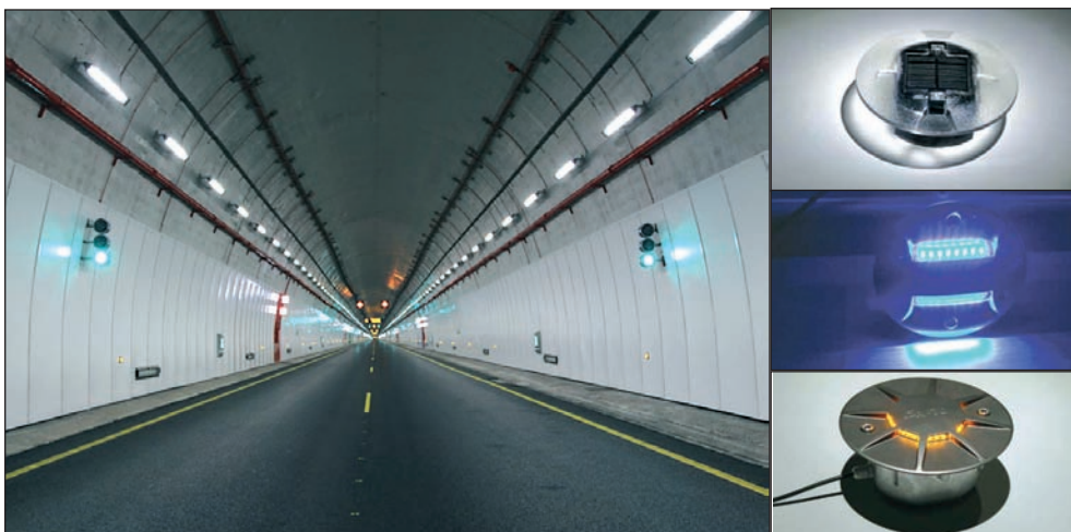
Túnel de O Folgoso, señalizado por Metrolight como parte de las obras de mejora en relación con la seguridad. A la izda. algunas de la luminarias para túneles y carreteras.
